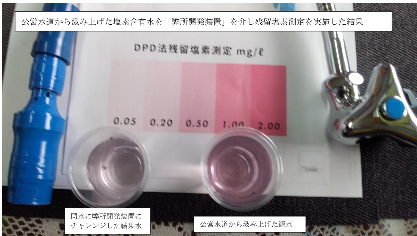
磁化水を介した曝気気泡装置での塩素除去結果 2
